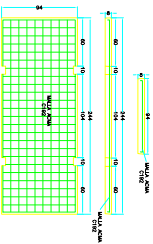
PLANTA TAPA 1:50
