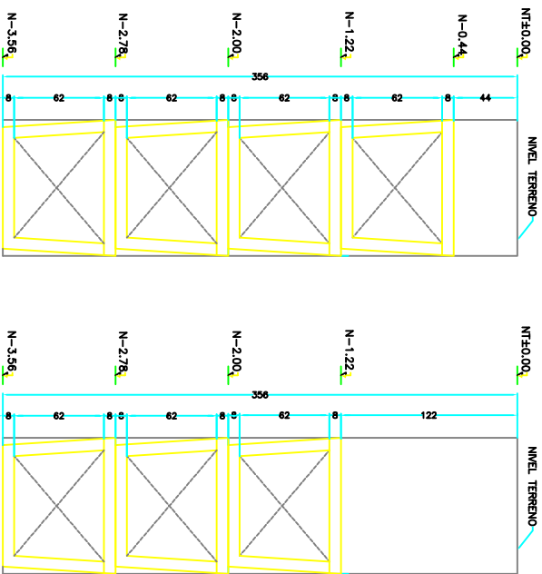
PROTECCION CUATRO SARCOFAGOS 1:50
